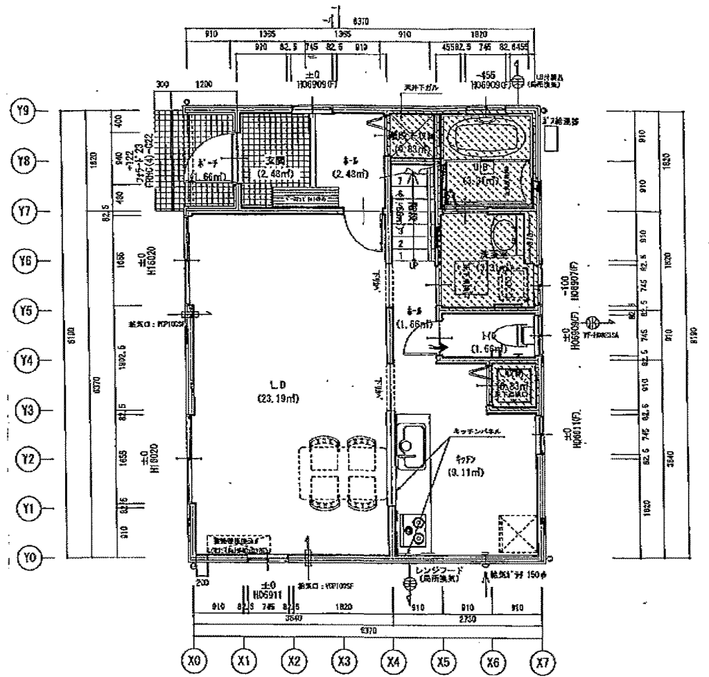
1階部分間取図
