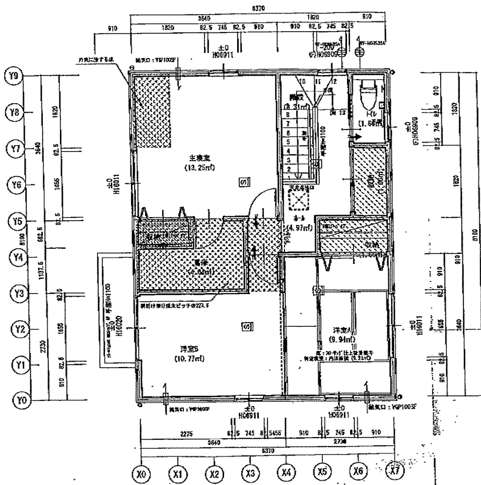
2階部分間取図
